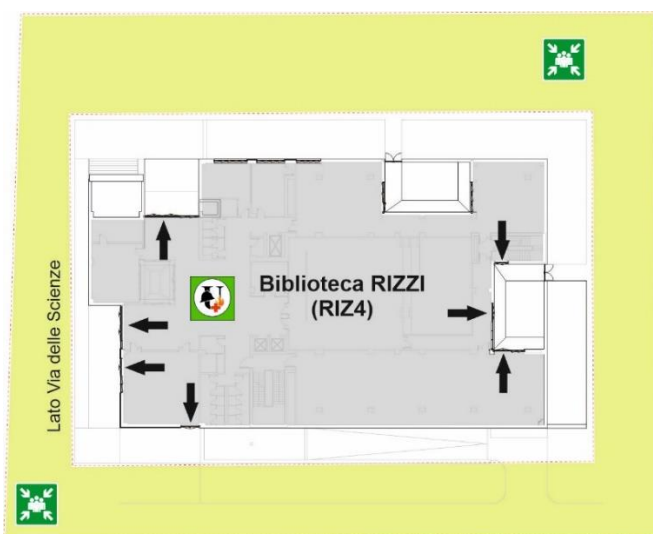
PLANIMETRIA - piano terra
